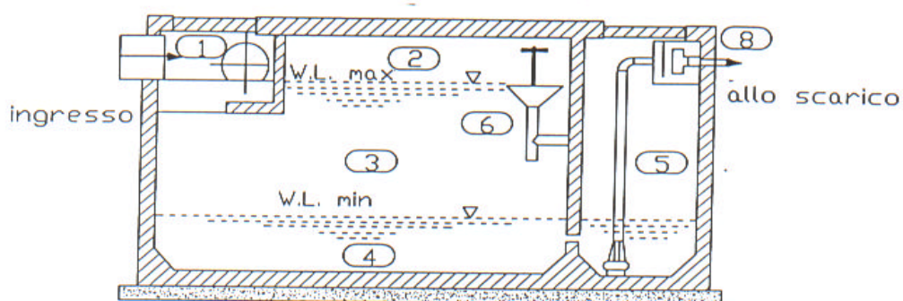
SCHEMA FUNZIONAMENTO VASCA DI PRIMA PIOGGIA
